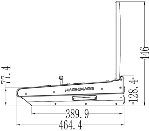
侧视图
