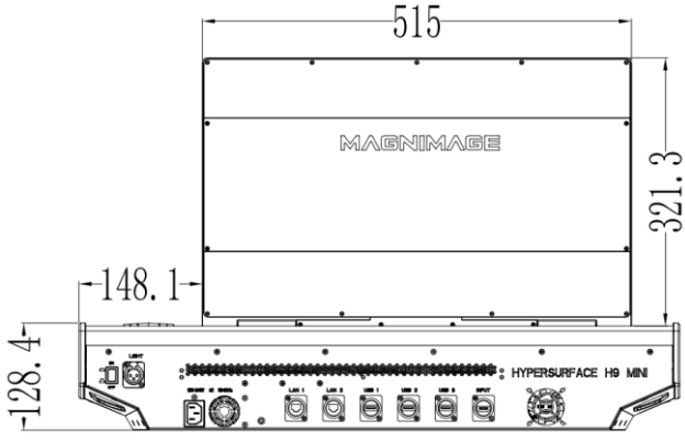
后视图
