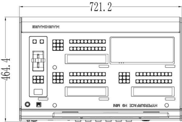
正视图
